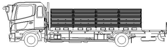
4t クラス(最大積載枚数 400枚)
